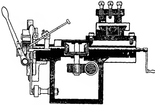
شكل 26 - مخرطة ويزورث (1835).
