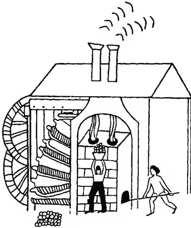
شكل 15. - مصمر عال. رسم إنكليزي من القرن السادس عشر.
