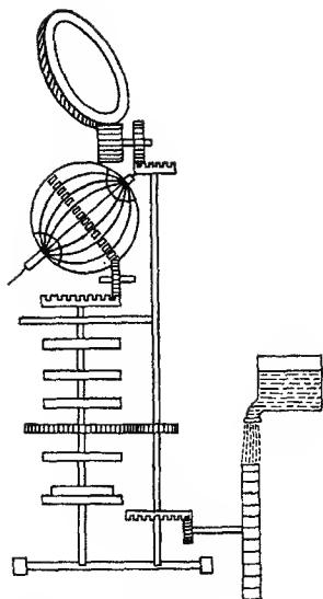
شكل 7. - ساعة فلكية (عن ج. نيد هام)
