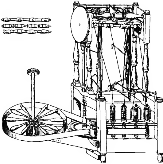
شكل 18 - آلة أركرايت Arkwright للغزل.
