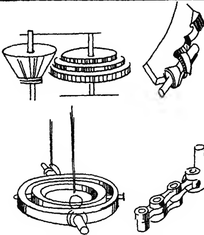
شكل 10. - مئلاج لتشبيكات (الموتاردو دافينشي).
