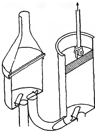
شكل 15. — مضخة كتيسبيروس الرافعة والدافعة (عن سوازي)
