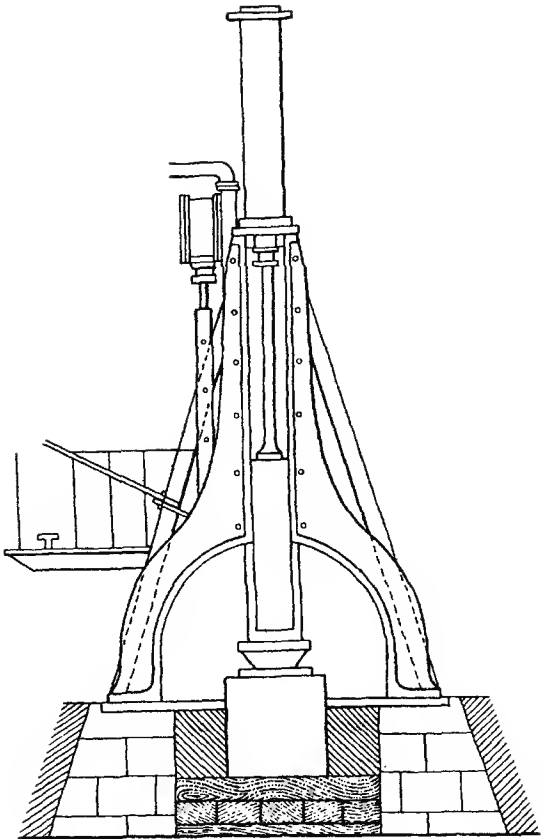
شكل 25 — أول مطرقة — هاون وضعها بوردون Bourdon.
