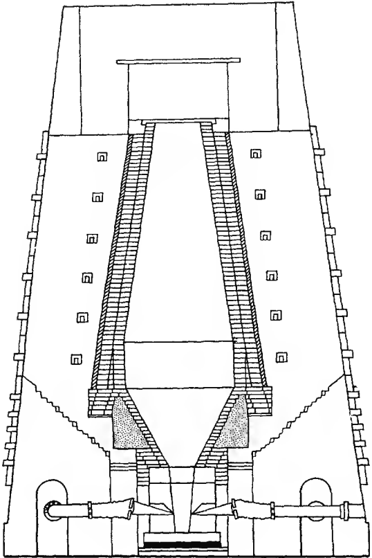
شكل 23 - مصرف غلوفيتز العالمي (سيليزيا (Silesie))، نحو سنة 1830.
