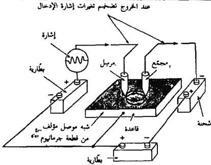
شكل 12 . الترانزستور الاتصالي مضخم الإشارات. (عن ص. هاندل).
