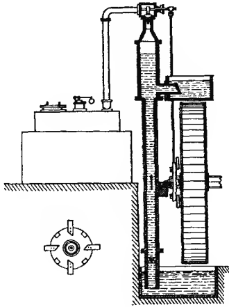
شكل 5 — آلة سافري Savery بعد أن حسنها كبير Kier ووريلي Wrigley.
