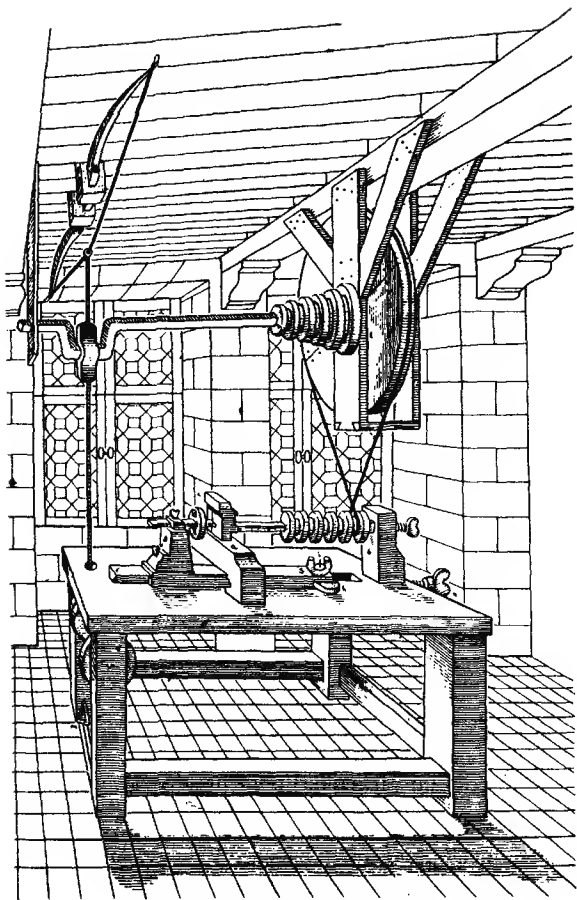
شكل 20. — مخروطة متغيرة السرعة (شبرويان، Chérubin، 1671).
