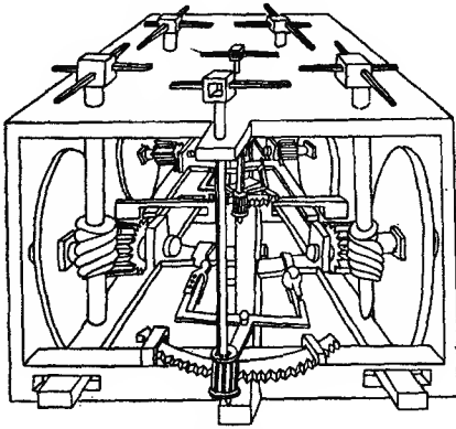
شكل 8 - العربة المتحركة بذاتها من فرنسيسكو دي جيورجيو.
