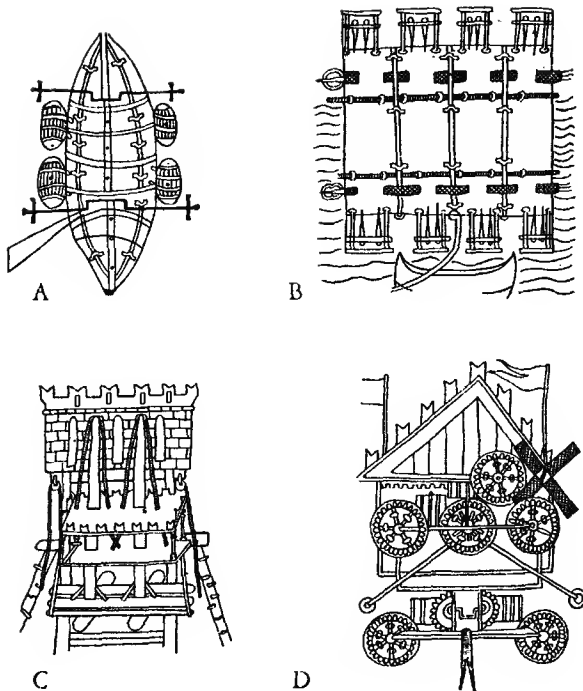
شكل ١. - آلات عمي دو فيجيدونو (نحو العام 1327). أ، الفواصة؛ ب، الجسر الخشبي؛ ج، برج الهجوم متغير الارتفاع؛ د، عربة دافعة هوائية.
