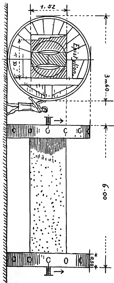
شكل 7. - جهاز نقل كتل حجرية في ايفيسوس. (عن بتروريوس).
