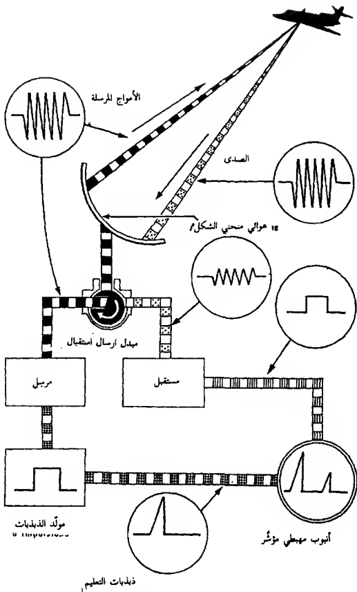
شكل 11 - تصميم الرادار (عن ص. هاننل).
