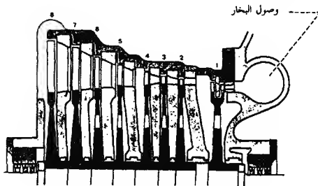
شكل 13 - ترتيبة متعدّدة الخلايا (راتو Rateau) ثمانى طبقات للضغط وتتضمن الأولى طبقتين للسرعة
