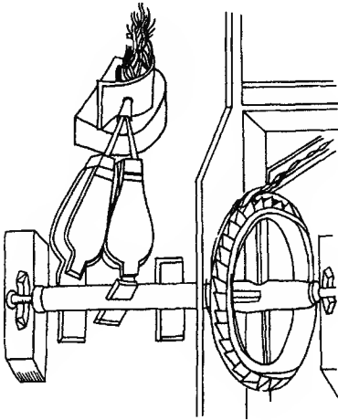
شكل 14. - مفاخ مائية (تاكولا).
