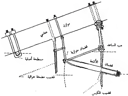
شكل 8 - متوازي الأضلاع المفصلي.
