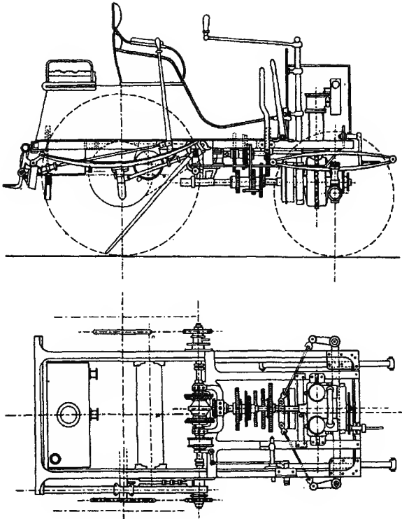
شكل 11 - التنظيم الميكانيكي الشامل لكلمبة بانهار Panhard ولوفاسور Levassor (1991 - 1994). Lvassor المحرك ذو اسطوانتين على شكل ضيق وقوة 4 حصنة (اسطوانتان 80 / 120).
