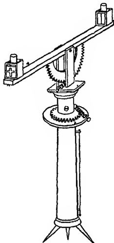
شكل 16. — كاسير الضوء عند هارون الاسكندراني.
