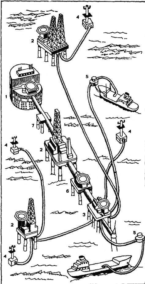
شكل 1 - مجموعة إكوفيسك Ekofisk الصناعية. 1، مستودع تخزين 160000 م 3 ، 2، مسطحات الحفر الثلاث، 3، مسطحة المعالجة، 4، آبار في طور الاستثمار، 5، طوافتان للتحميل، 6، أبديّة سكنية، 7، مسطحة للضخ. (عن رسم إ. ف. فيزان Ph. Ferran ورد في جريدة «الموند»).
