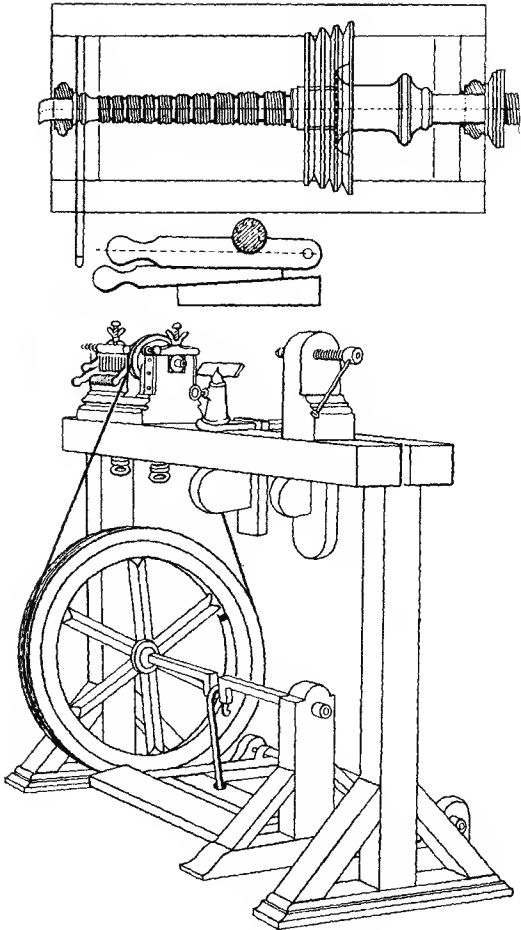
شكل 1 - مخرطة للنحت (1785).
