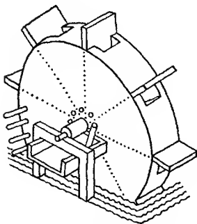
شكل 7. - عجلات رافعة مرسمة (عن شوازي Choisy «Vitruve»).
