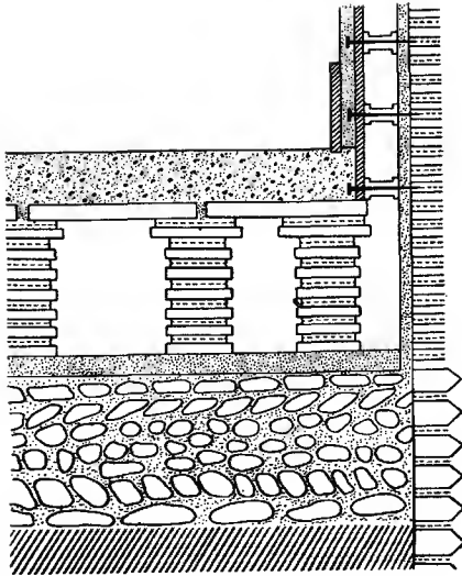
شكل 17 - مقطع من فون لرضي قديم. (عن م. دوما)
