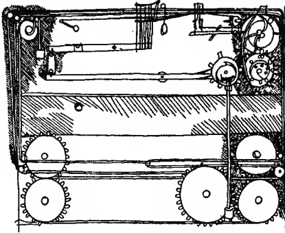
شكل 24. - آلة نسيج أوتوماتيكية (الموناردو داهينشي).
