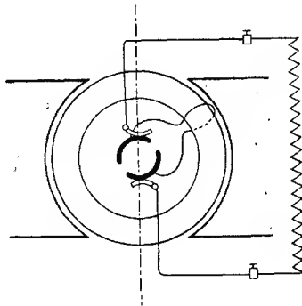
شكل 9 - مبدأ الدينامو (عن ليبر Lehr)
