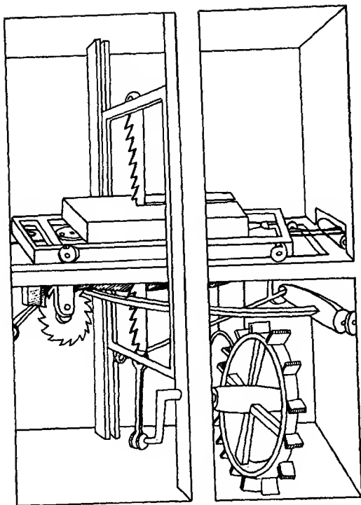
شکل 17. - منشار ماني (فرزشسکو دي جهورجيو).
