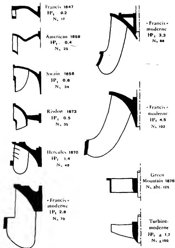
شكل 3 — التطور الذي طرأ على شكل ريش التربينات (عن مانتر Hunter، « Les Origines des turbines Francis et Pelton » مجلة تاريخ العلوم، باريس، 1964).
