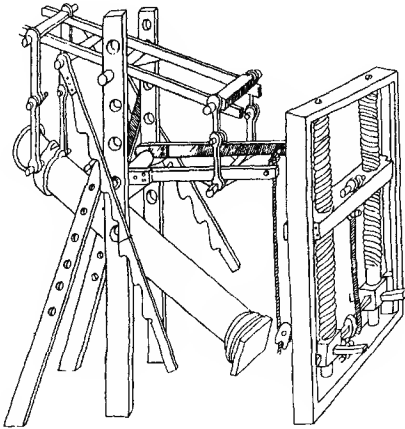
شكل 30. — اجهزة الرفع لدى فرنسيسكو دي جيورجيو.
