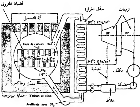
شكل 2 - تصميمه مركز الأورانيوم الطبيعي هينكلي بونت Hinkley Point. (م. ج. بارين Les Centrales nucléaires, G. Parreins, باريس، 1967).
