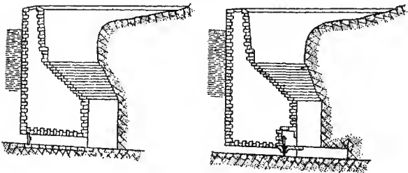
شکل 28. — مقطع و ارتفاع حاجز المانسا Almansa (نحو 1550-1560).
