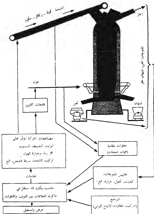
شكل 15 - مخطط نظري لتألية فرن عال شاملة.
