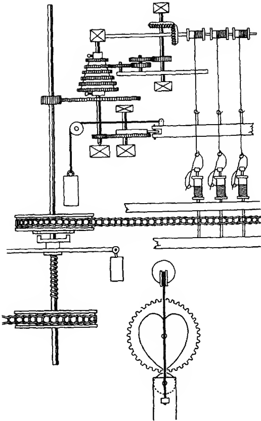
شكل 20 — أجهزۃ التوجيه في مجالل فوكانسون للحريز. (عن دوانون Doyon ولديهفتر Liaigre).
