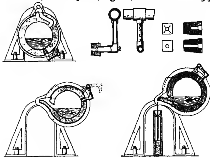
شكل 10 - محوّل بسمر Bessemer عن براءة سنة 1855
