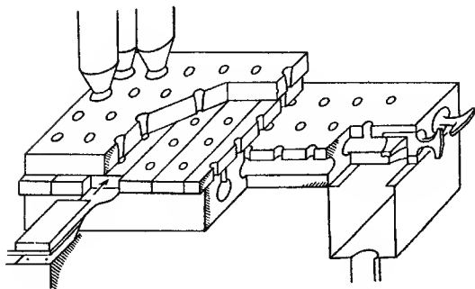
شکل ۱۴ - متناخ مائیه (ارغن)
