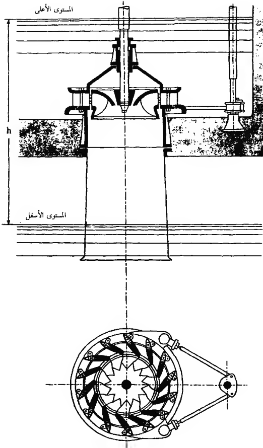
شكل 1 — توربينة فرانسيس Francis (عن لير Lehr, « Les Moteurs », باريس، 1970)
