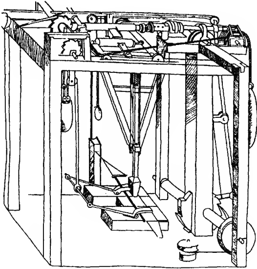
شكل 16. - مطرقة للقطع الكبيرة (البوناردو دافينشي)
