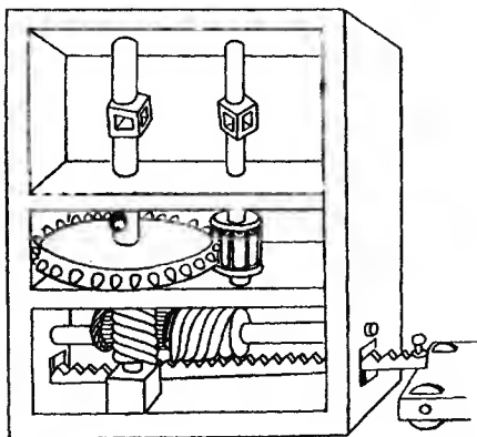
شكل 11. - استعمال اللولب غير المتطهي (فرنشسكو دي جيورجيو).
