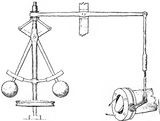
شكل 9 - الضابط ذو الكرات.
