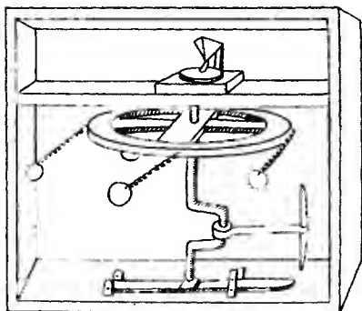
شكل 12. - اول محاولة للضبط (فرنشسكو دي جيورجيو).
