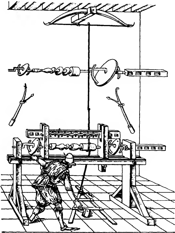
شكل 18. - مخروطة عن ج. هيشون (1878).
