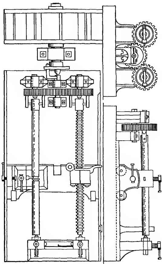
شكل 2 - مخرطة الخشب (1798).
