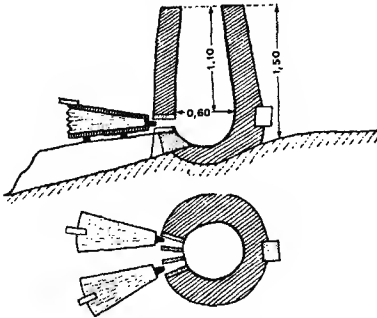
شكل 9. فرن لانترومال (منطقة السار)
